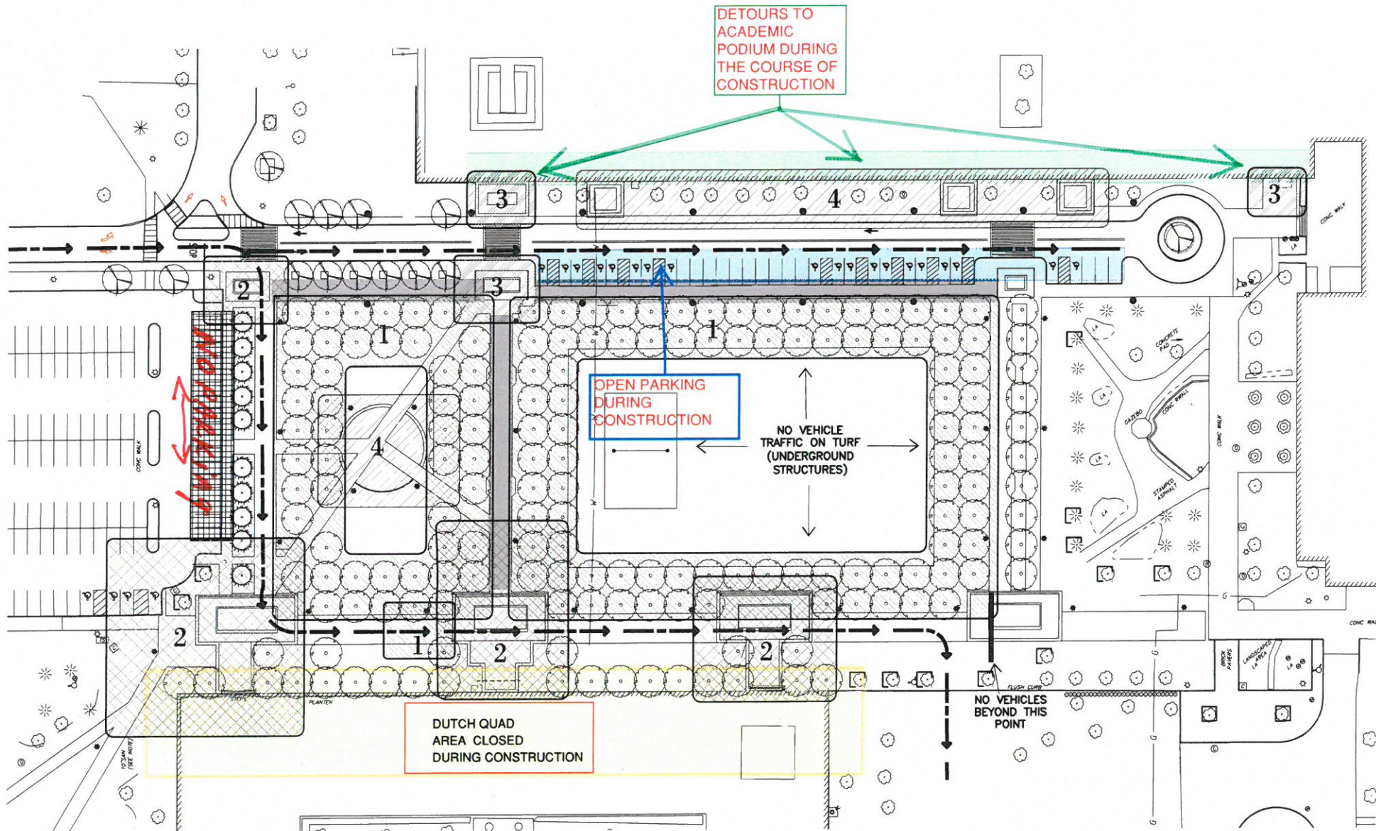
STAGING PLAN 2017 DUTCH COMMONS PROJECT
